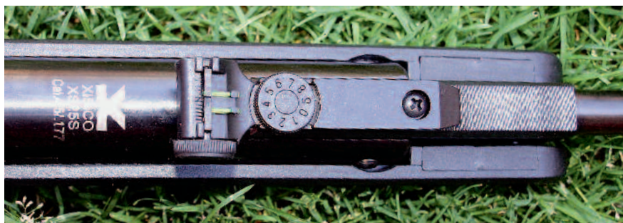
Hledí je výškově i stranově stavitelné, po stranách orámované světlovednými vlákny
