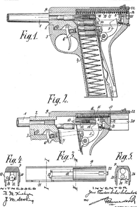
Patentová skica pistole amerického patentu č. 733681 ze 14. 7. 1903
