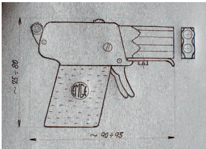
◀ Náčrt pistole po 65 letech
