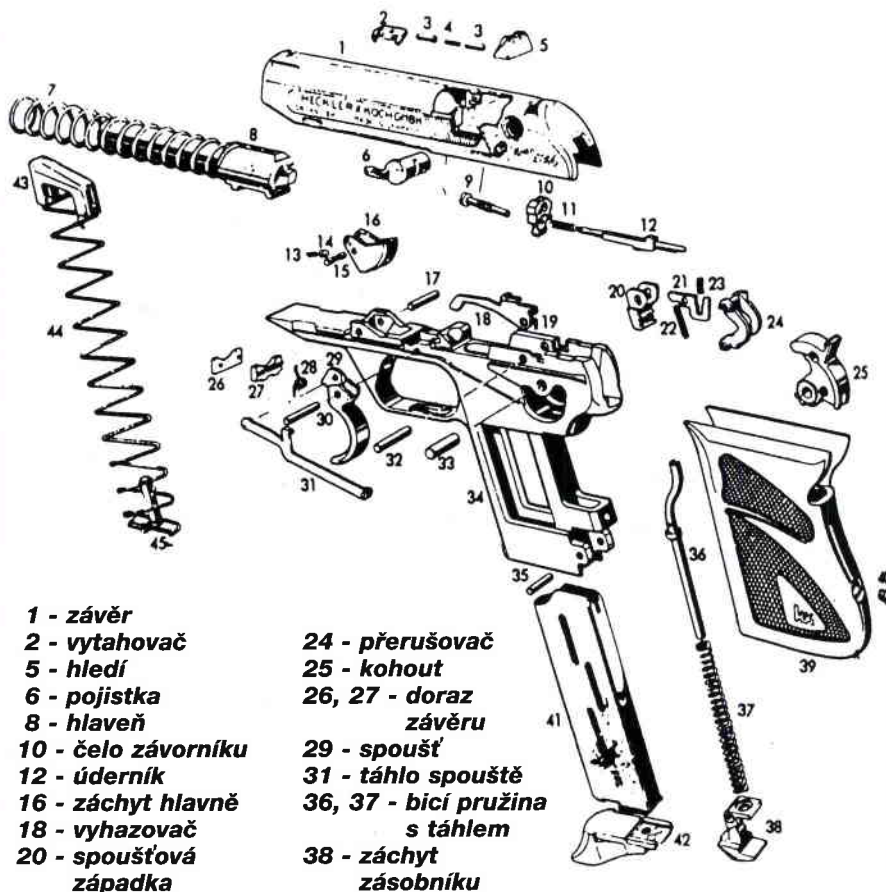
HK 4 (popsány pouze hlavní součásti)
